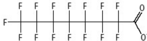
PFOA
