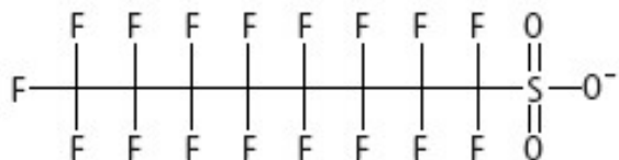
PFOS
